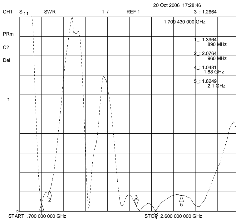
Joonis 3. Antenni sisendi SWR karakteristiku näidis
