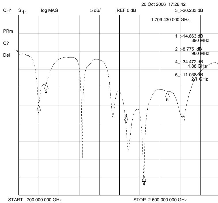
Joonis 2. Antenni sisendi S 11 karakteristiku näidis
