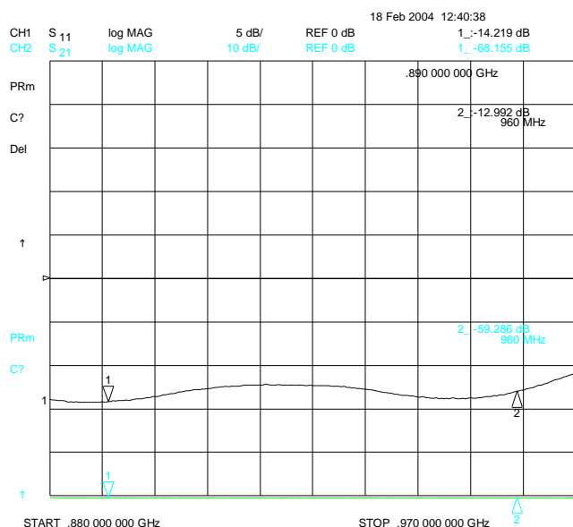
Joonis 1. Antenni sisendi S11 karakteristiku näidis
