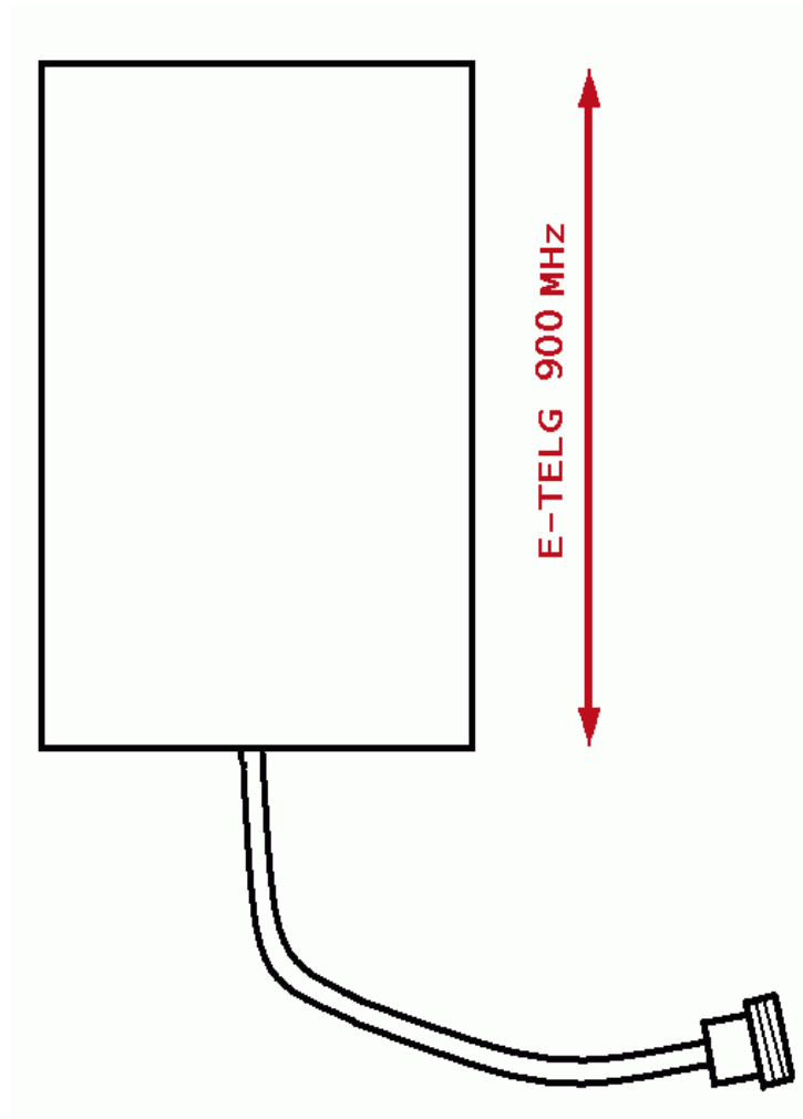
Joonis 2. Polarisatsioon
