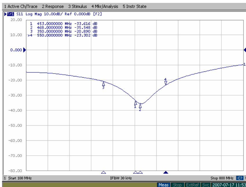
Joonis1. Tüüpiline sobituse (S11) karakteristik.
