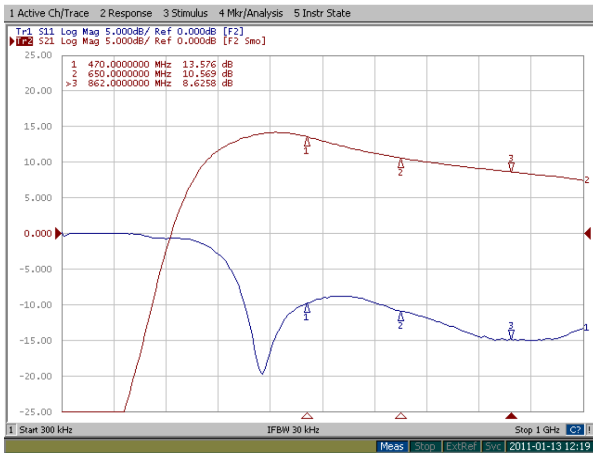
Joonis 1: Sobituse (S11) ja ülekanne (S21) karakteristikute näidised.
