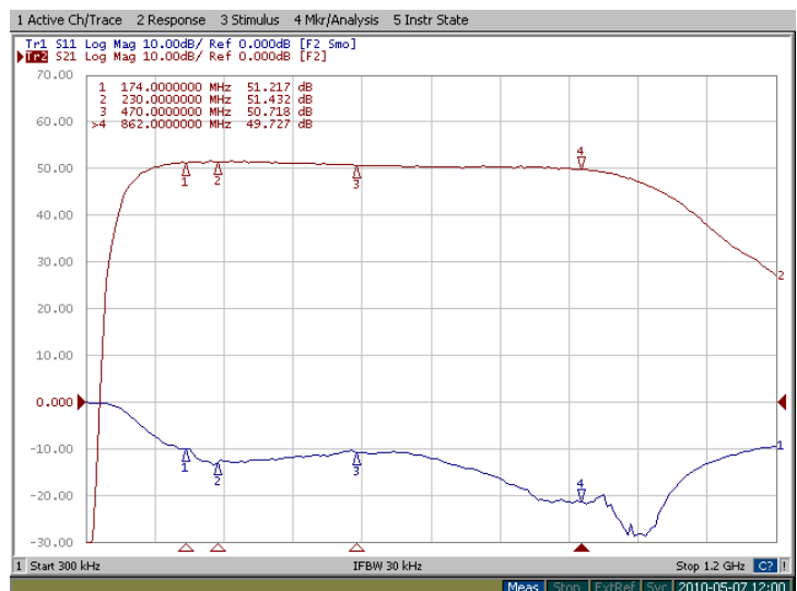
Sobituse (S11) ja ülekande (S21) karakteristikute näidis.
