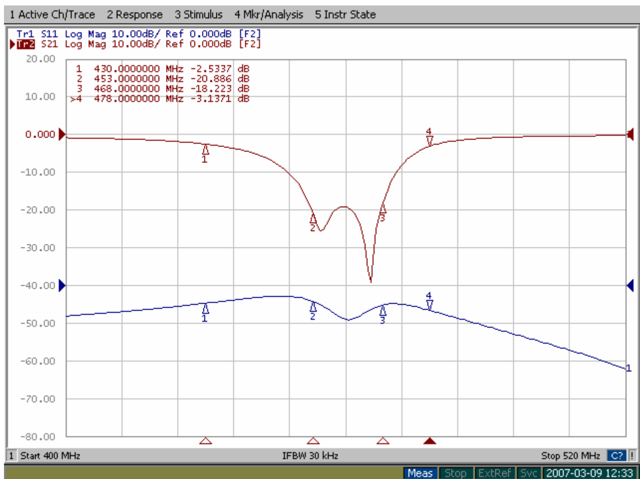
Joonis 1. Ülekandekarakteristik S21 ja sobitustegur S11; 400 - 520MHz
