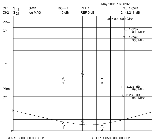
Joonis 1. Jaguri ülekanne ja sobituse (S 21 ja SWR) karakteristikute näidis
